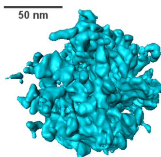
Reconstruction 3D d'un agrégat de cobalt (réduit) obtenu par tomographie électronique.
