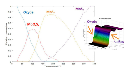
Évolution des spectres XANES et de la concentration relative des quatre espèces principales en fonction de la T° de sulfuration.
