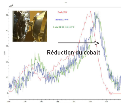
Chambre d'analyse et évolution du spectre Co 2p oxyde, après réduction sous 1 mbar \text{H}_2 400 °C et sous \text{H}_2:\text{CO} (2:1) à 230 °C.
